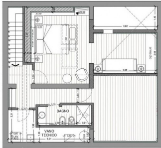
PIANO PRIMO
